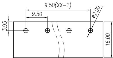
P.C.B. LAYOUT
