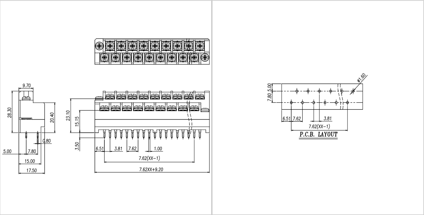
尺寸图
