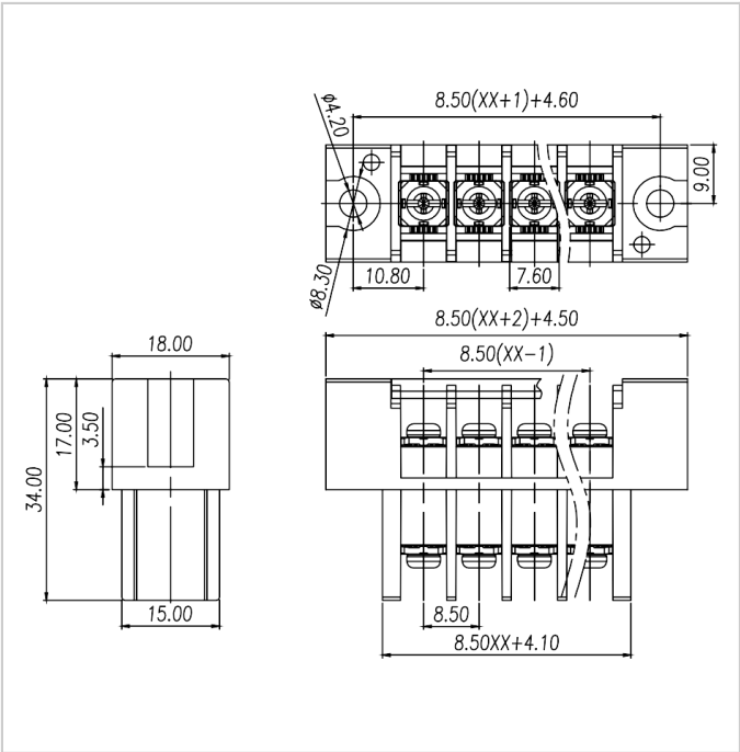
尺寸图
