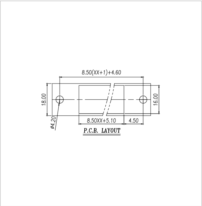
PCB开孔图
