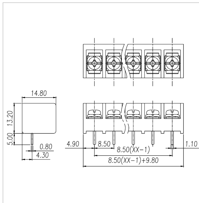
尺寸图
