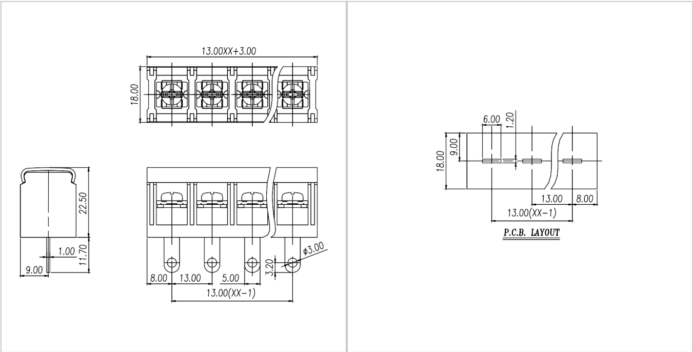
尺寸图
