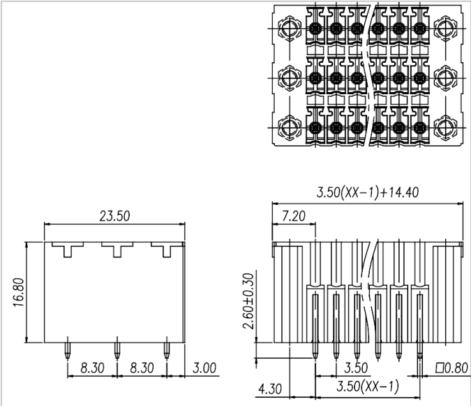
尺寸图
