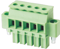
WJ15EDGKRN-3.5/3.81
