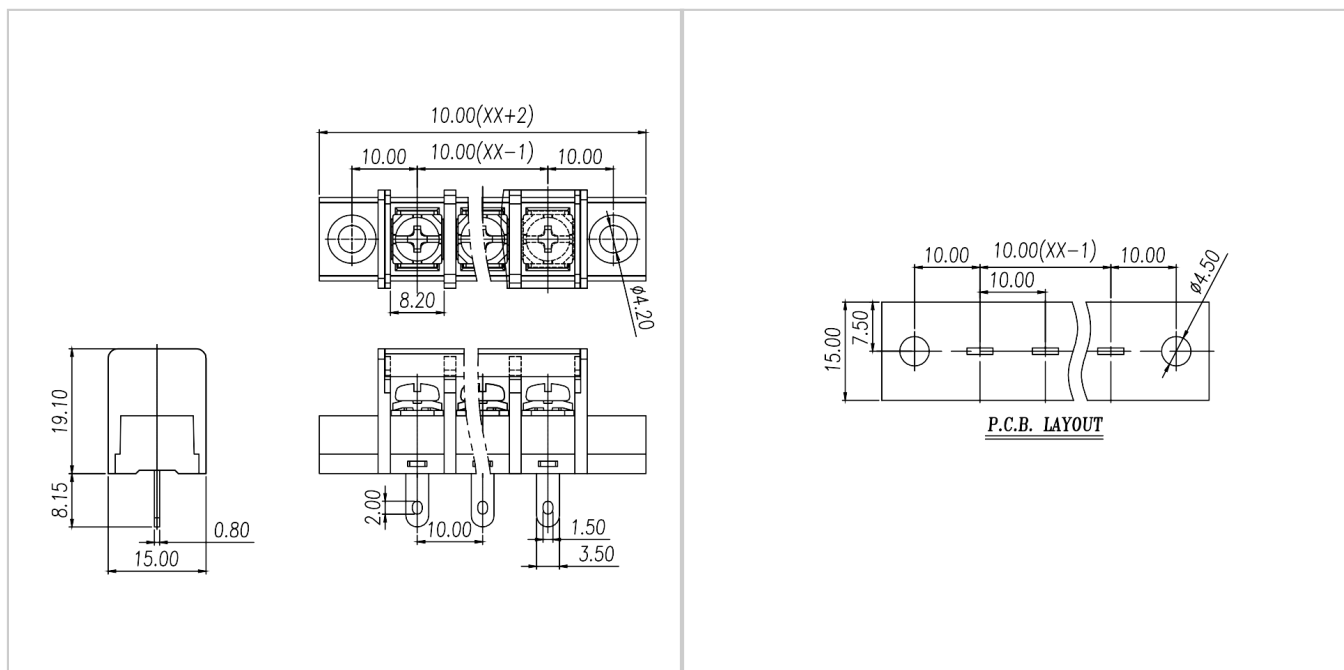
尺寸图
