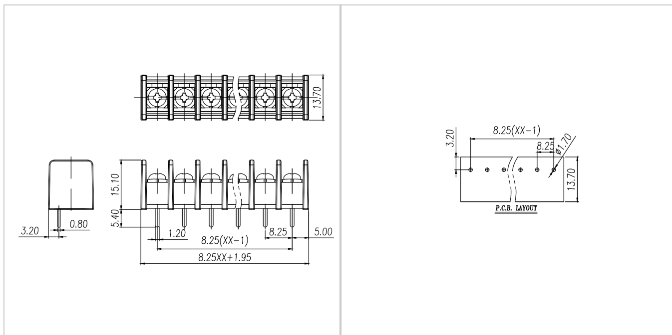
尺寸图
