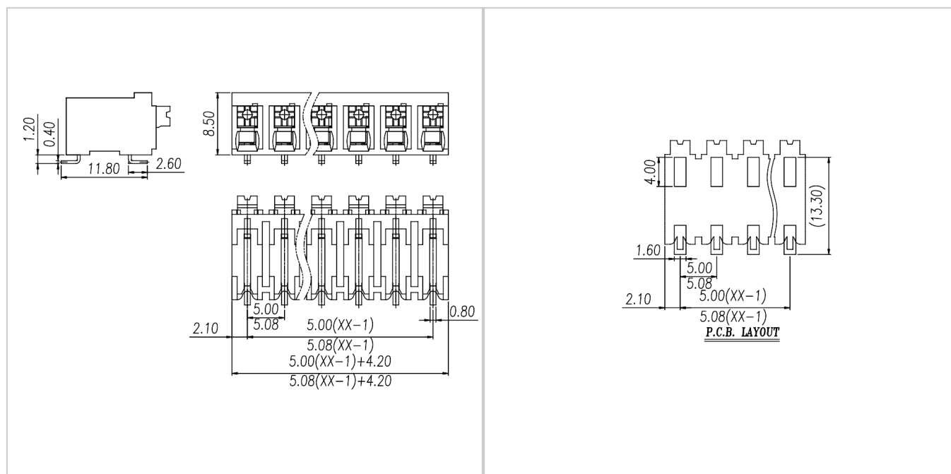
PCB开孔图
