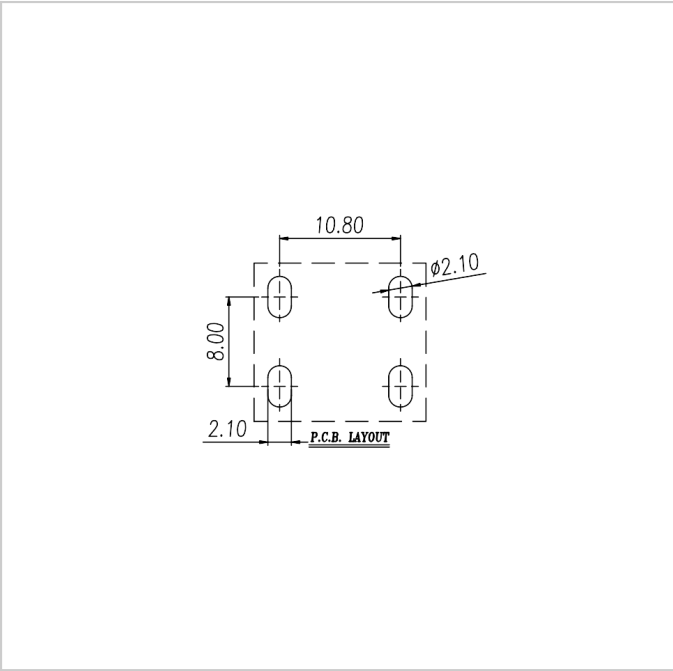
PCB开孔图
