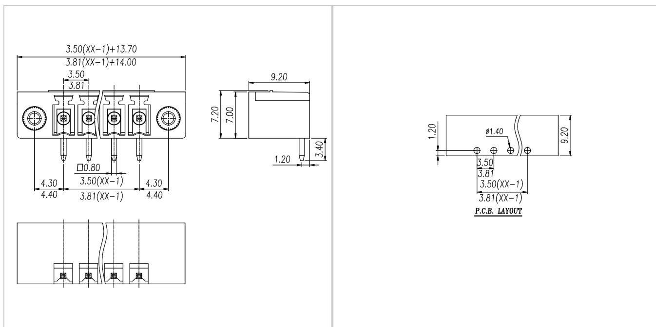
配件
