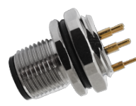
M12 公头面板式，PCB型，后锁安装， 屏蔽针
