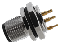
M12 公头面板式，PCB型，后锁安装， 屏蔽针
